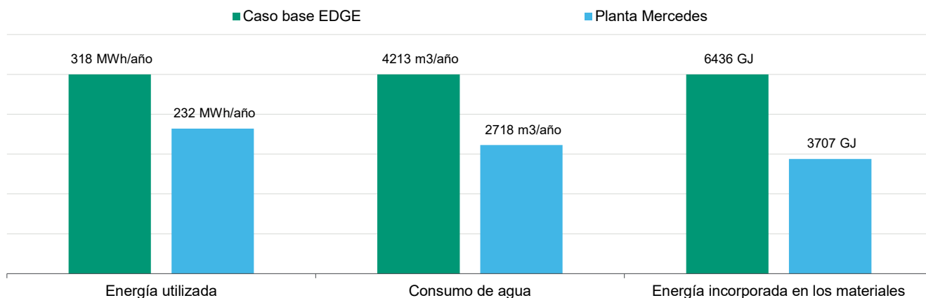
Figura 1: Utilización de energía, agua y energía incorporada en los materiales del Proyecto Mercedes Tecnovax
